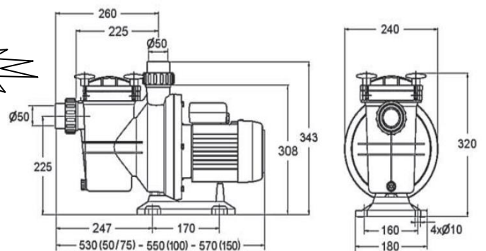
Dimensiones / Dimensions (mm)
